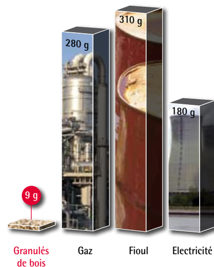
Emissions de CO 2 en g/kWh
